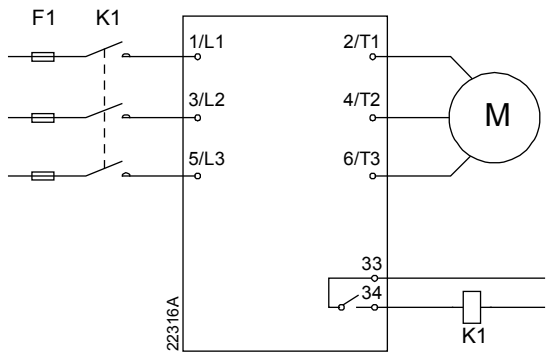
装有主接触器的软起动器
