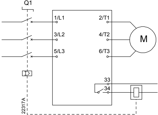
装有分流继电器和断路器的软起动器
